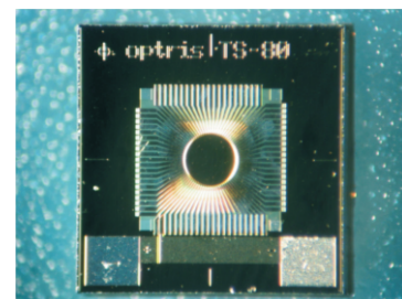
Thermosäule TS80
