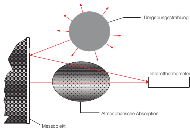
Umgebungsstrahlungskompensation
