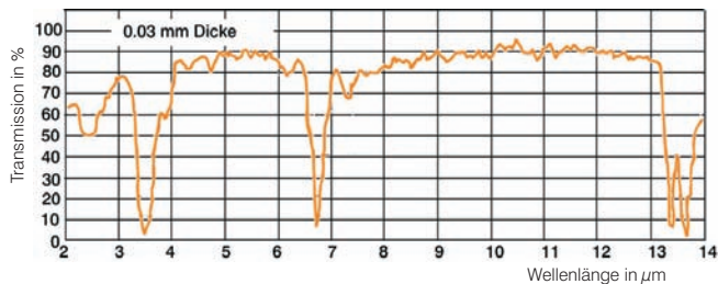
Spektrale Durchlässigkeit von Kunststoffolien aus Polyester
