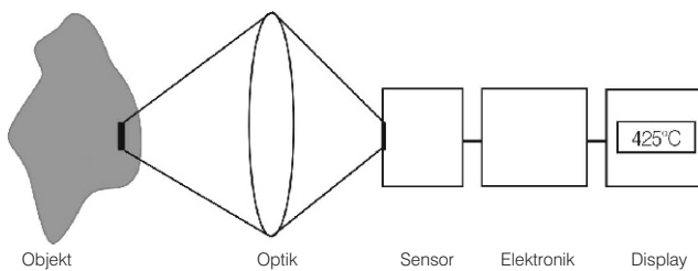
Infrarotsystem
