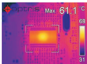
Temperaturmessung an einem Schaltkreis mit Hilfe der Maximalwertfunktion
